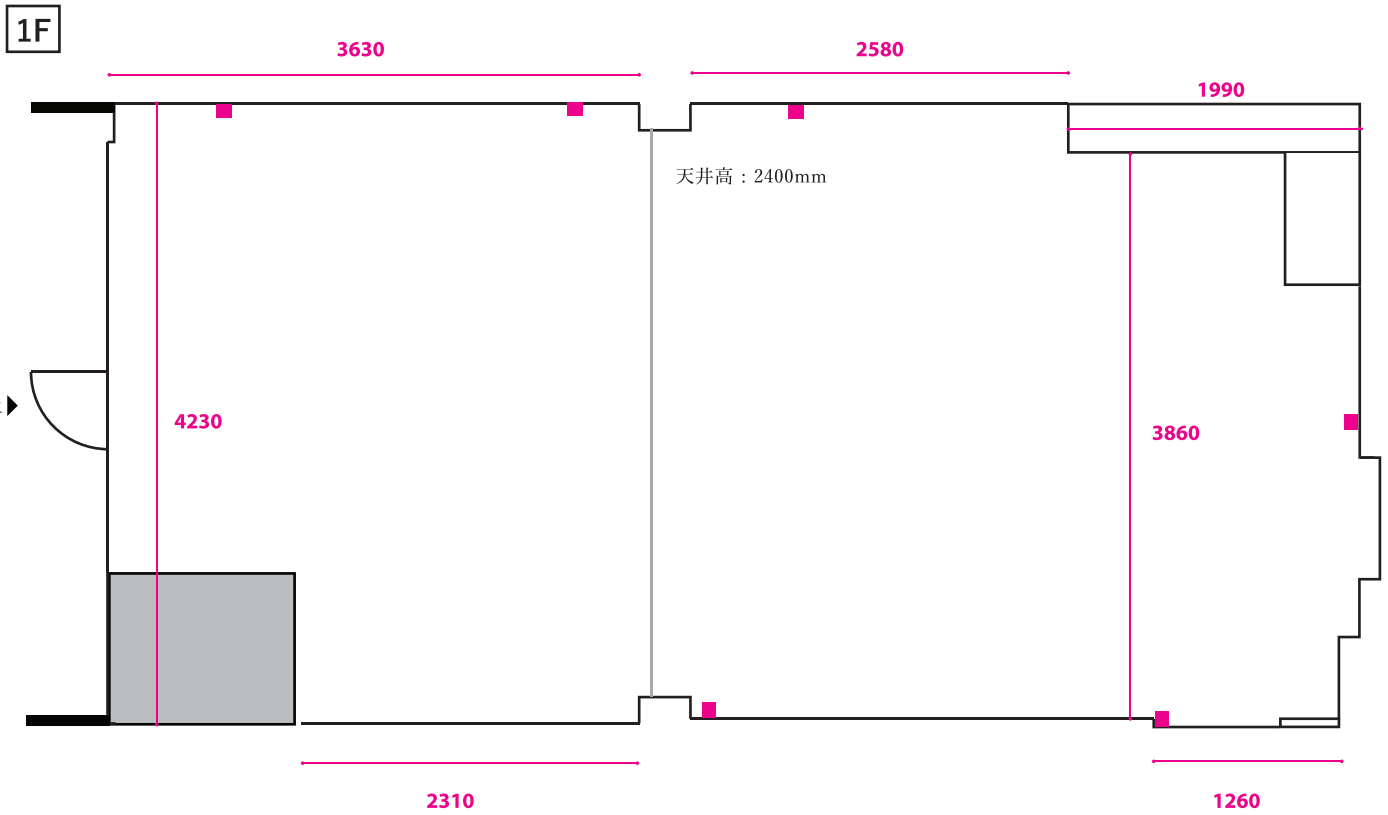
平面図
